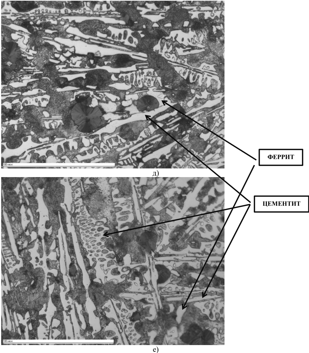
Рис. 5. Микроструктура матрицы чугунов, \times 400 , травлено, модифицированных: а) лигатурой M21, б) лигатурой M22
