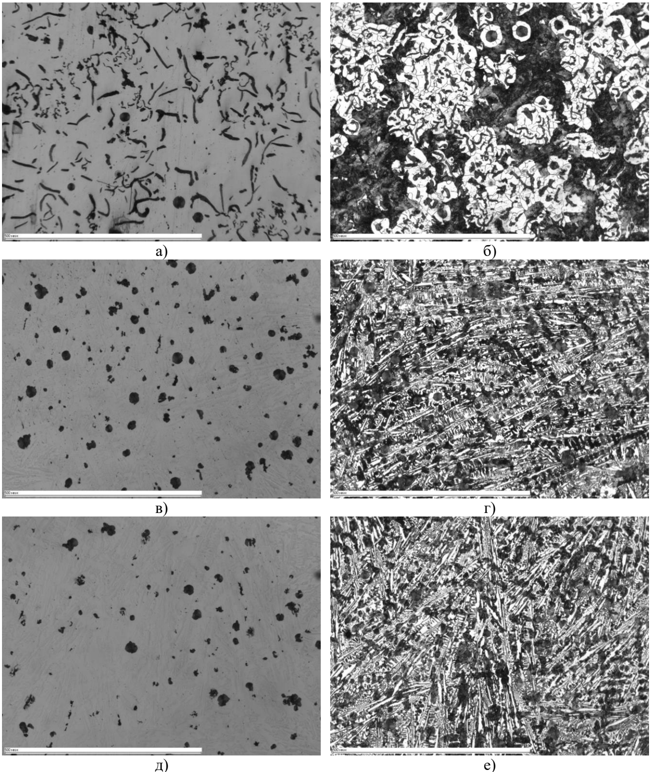
Рис. 4. Микроструктура чугунов, модифицированных опытными лигатурами: а,б) M13, в,г) M21, д,е) M22, соответственно а,в,д) \times 100 , не травлено, б,г,е) \times 400 , травлено
